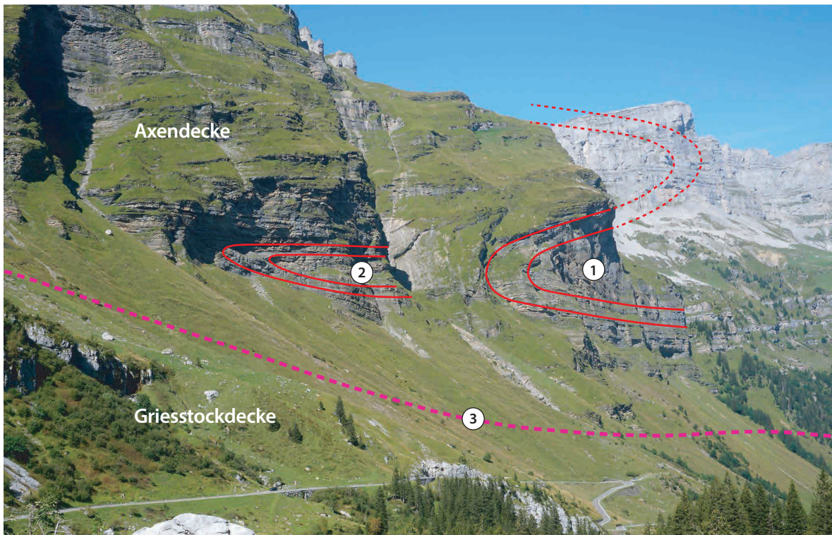
Abb. 3: Falte in den Sedimentschichten der Unteren Jurazeit auf der Nordseite der „Chlus“ (rot nachgezeichnet). Es fällt auf, dass die Falte in „steifen“, sogenannten kompetenten Schichten (1) offener ist als in „weichen“, sogenannten inkompetenten Schichten (2). Die violett gestrichelte Linie (3) markiert den vermuteten Verlauf der Deckengrenze zwischen Griesstock- und Axendecke unter dem Schutt.
