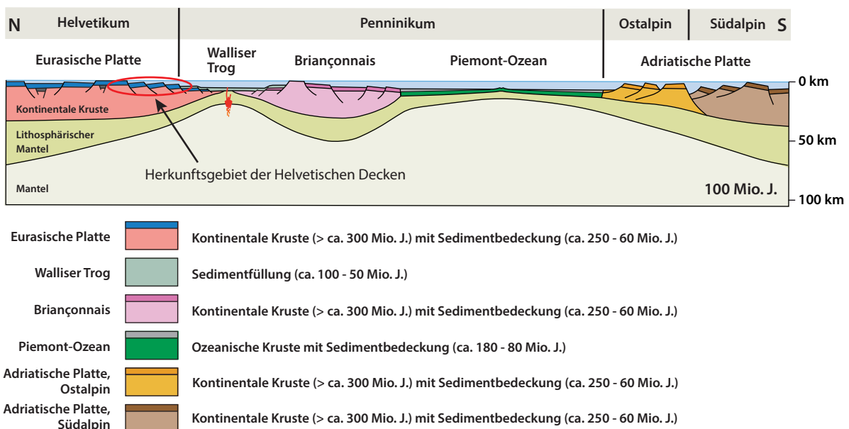
Abb. 4: Die sechs tektonischen Einheiten, welche später die Alpen aufbauen werden. Die Helvetischen Decken stammen vom südlichen Rand der Eurasischen Platte (siehe auch Modul 5, Abb. 5 ).
