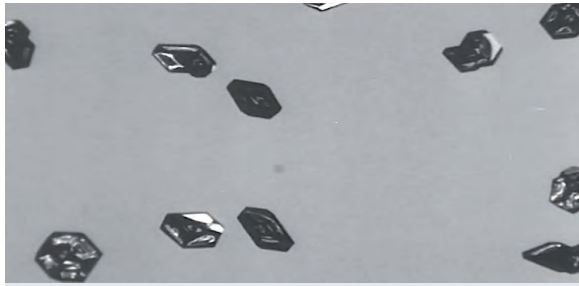
A: Kristallwachstum in einer Schmelze im Labor.
