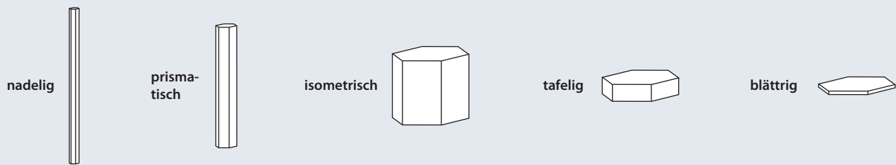
Abb. 5: Gebräuchliche Habiti (Sg. Habitus) am Beispiel eines hexagonalen Prismas. Auch jede andere Kristallform kann unterschiedliche Habiti haben.
