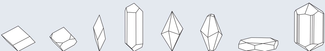
Abb. 4: Formenvielfalt der Kalzitkristalle.
