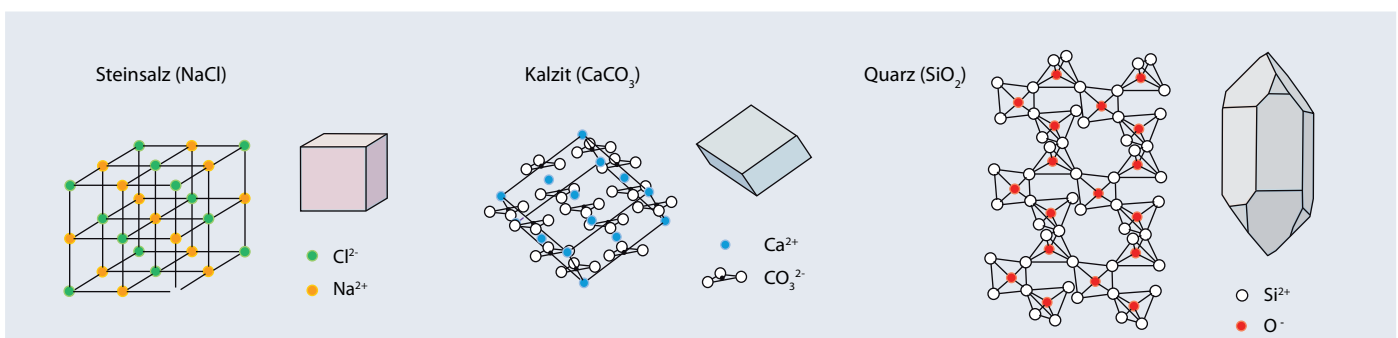
Abb. 1: Kristallgitter und ideale Kristalle
