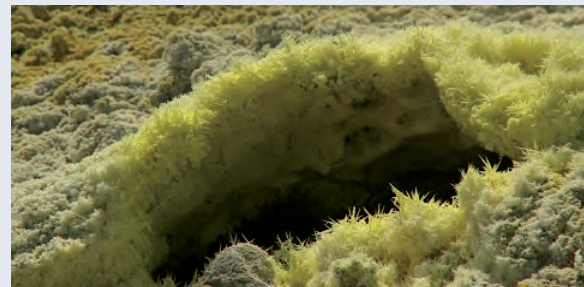
D: filigrane Schwefelkristalle, die an einem Vulkan aus heißen Gasen resublimieren.
