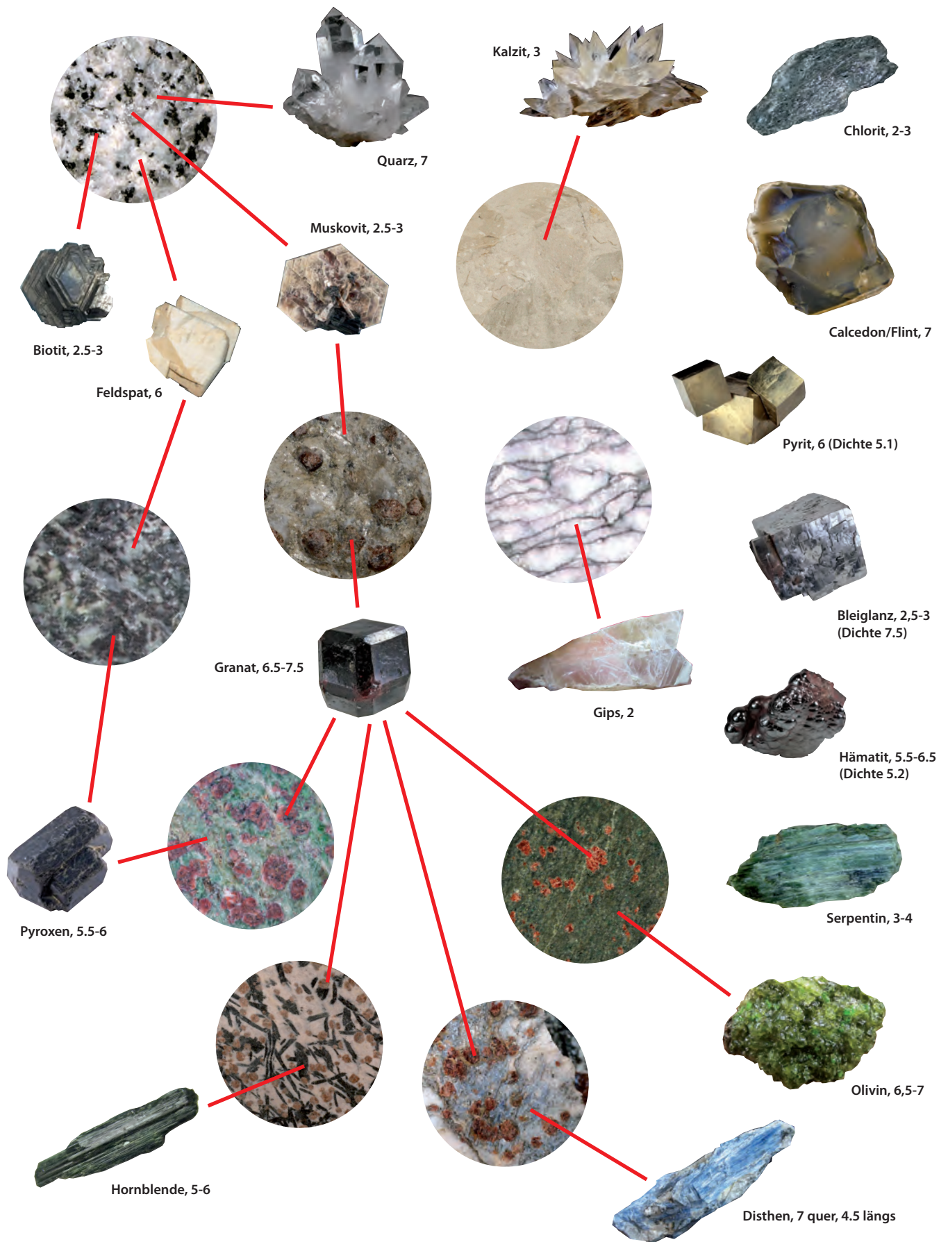
Abb. 7: Minerale einzeln und im Gesteinsverband, mit jeweiliger Ritzhärte. Disthen ist längs weicher als quer; die drei Erze Pyrit, Hämatit und Bleiglanz haben eine hohe Dichte und sind deshalb besonders schwer.
